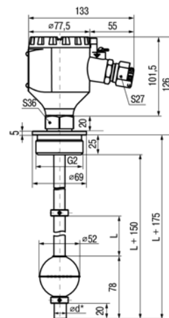
Рисунок 6.1 – Габаритные и присоединительные размеры
